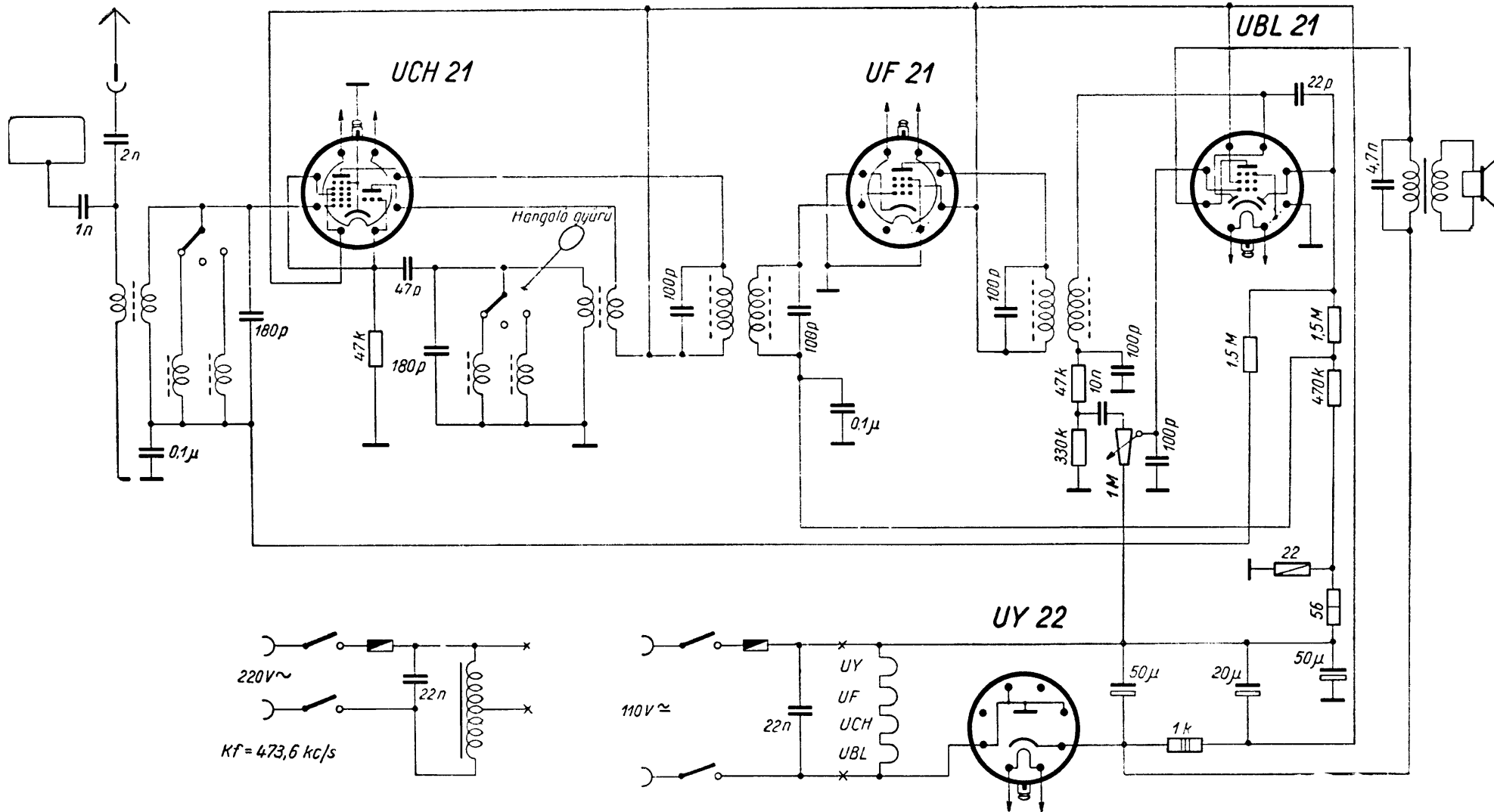
Orion 313 és Telefunken 313 NR
